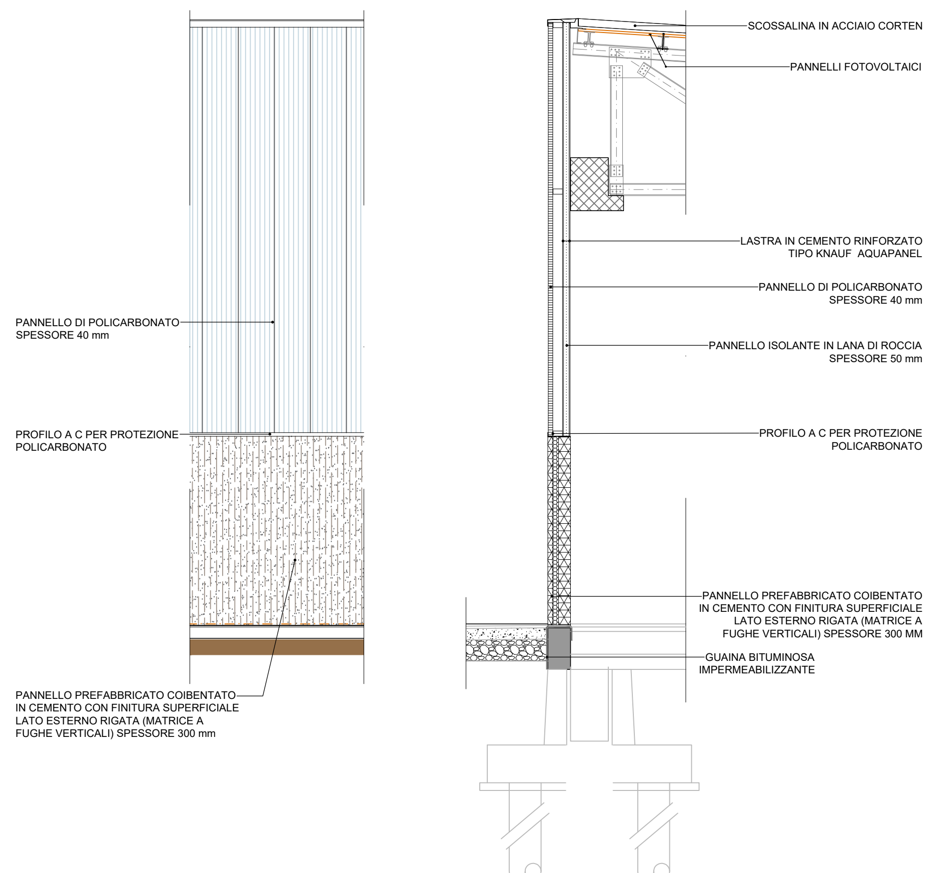
Dettaglio prospetto - sezione - scala 1:50
