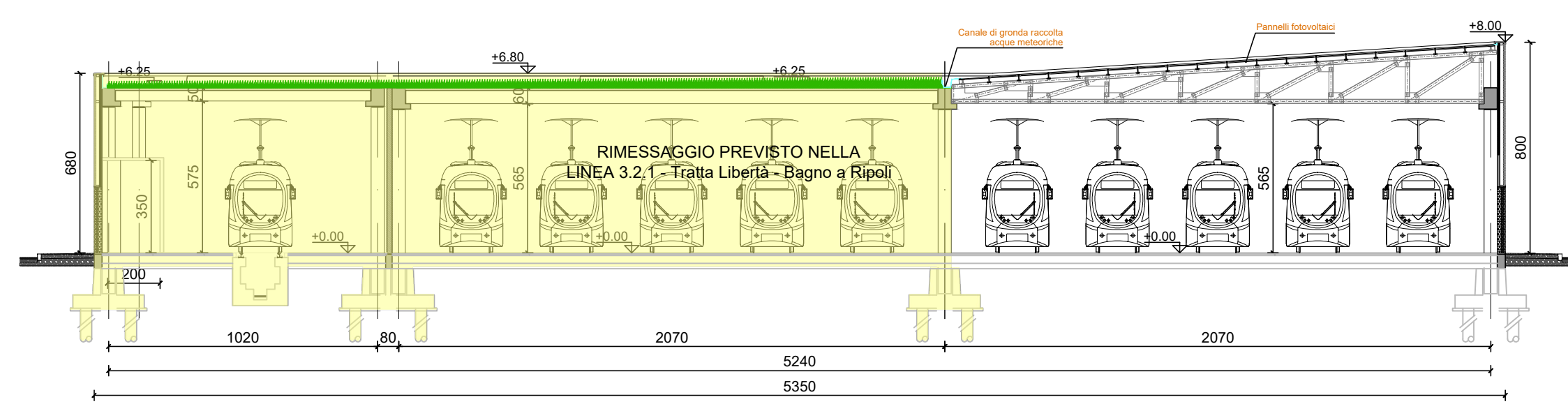
Sezione trasversale - scala 1:200
