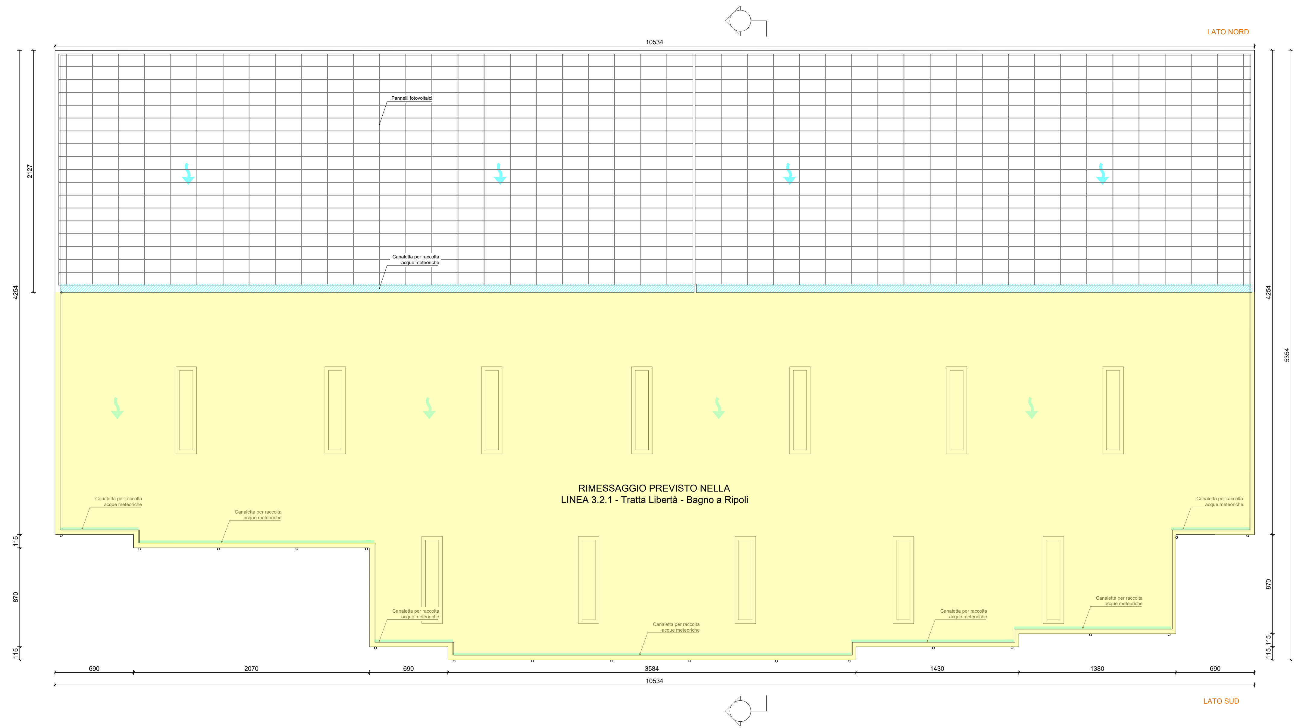
Pianta copertura - scala 1:200
