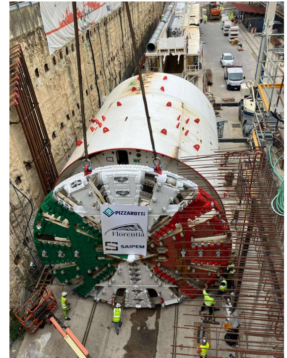
Seconda TBM per lo scavo della galleria Binario Dispari
