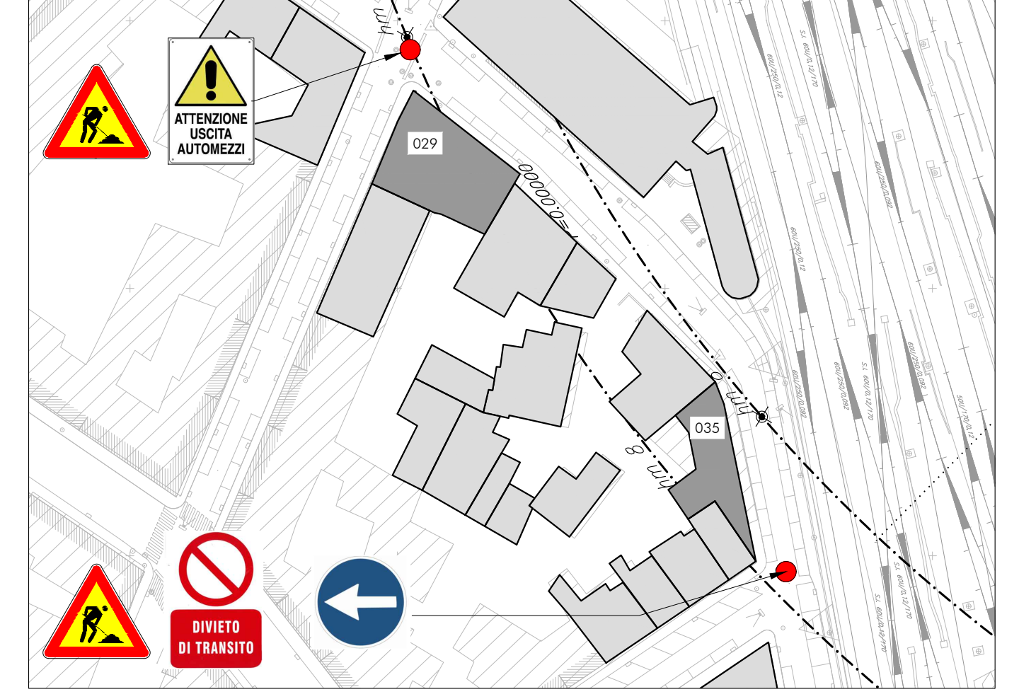
PLANIMETRIA DI INQUADRAMENTO scala 1:1000
