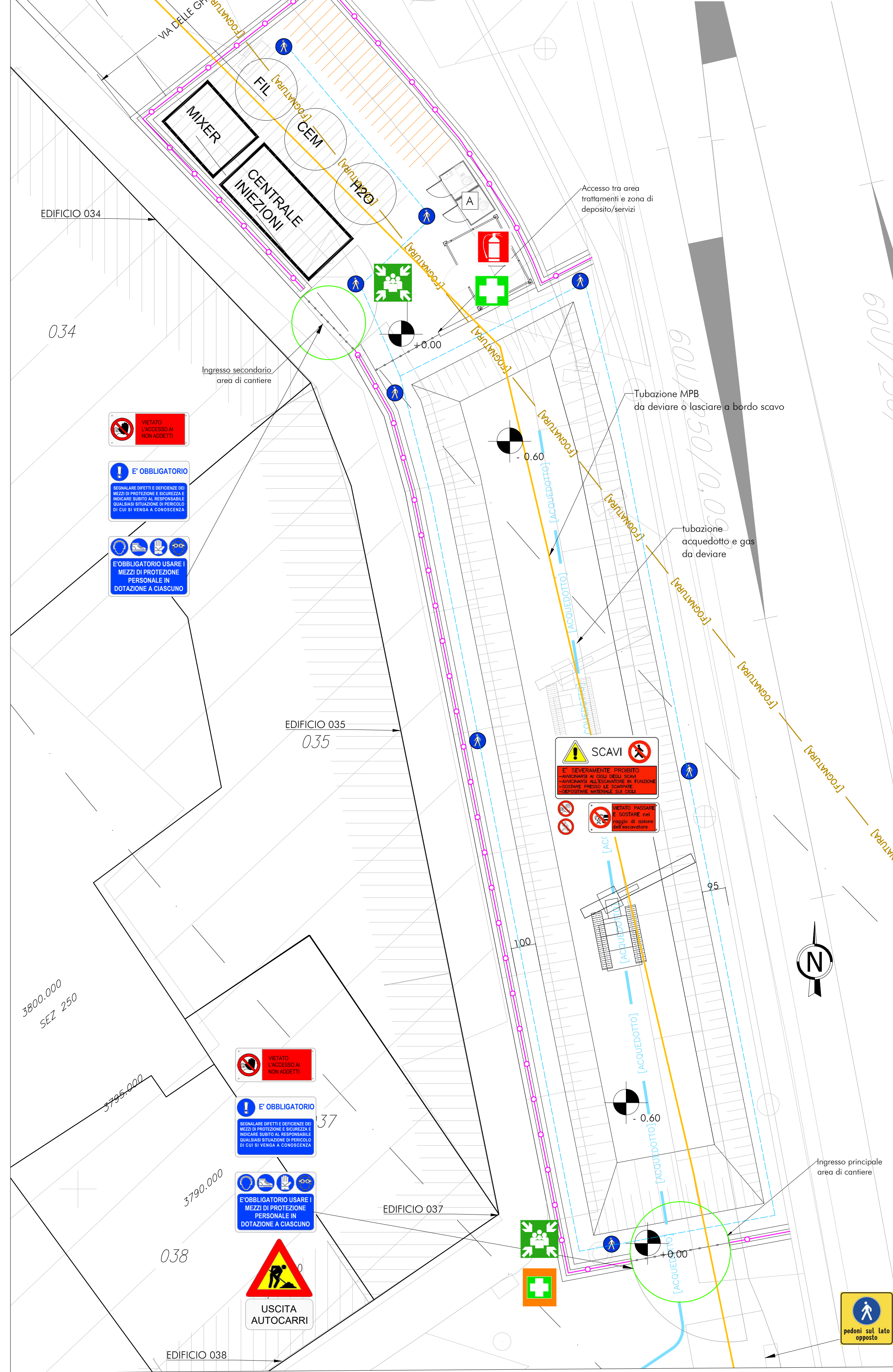
PLANIMETRIA LAYOUT CANTIERE - EDIFICIO 35 scala 1:200
