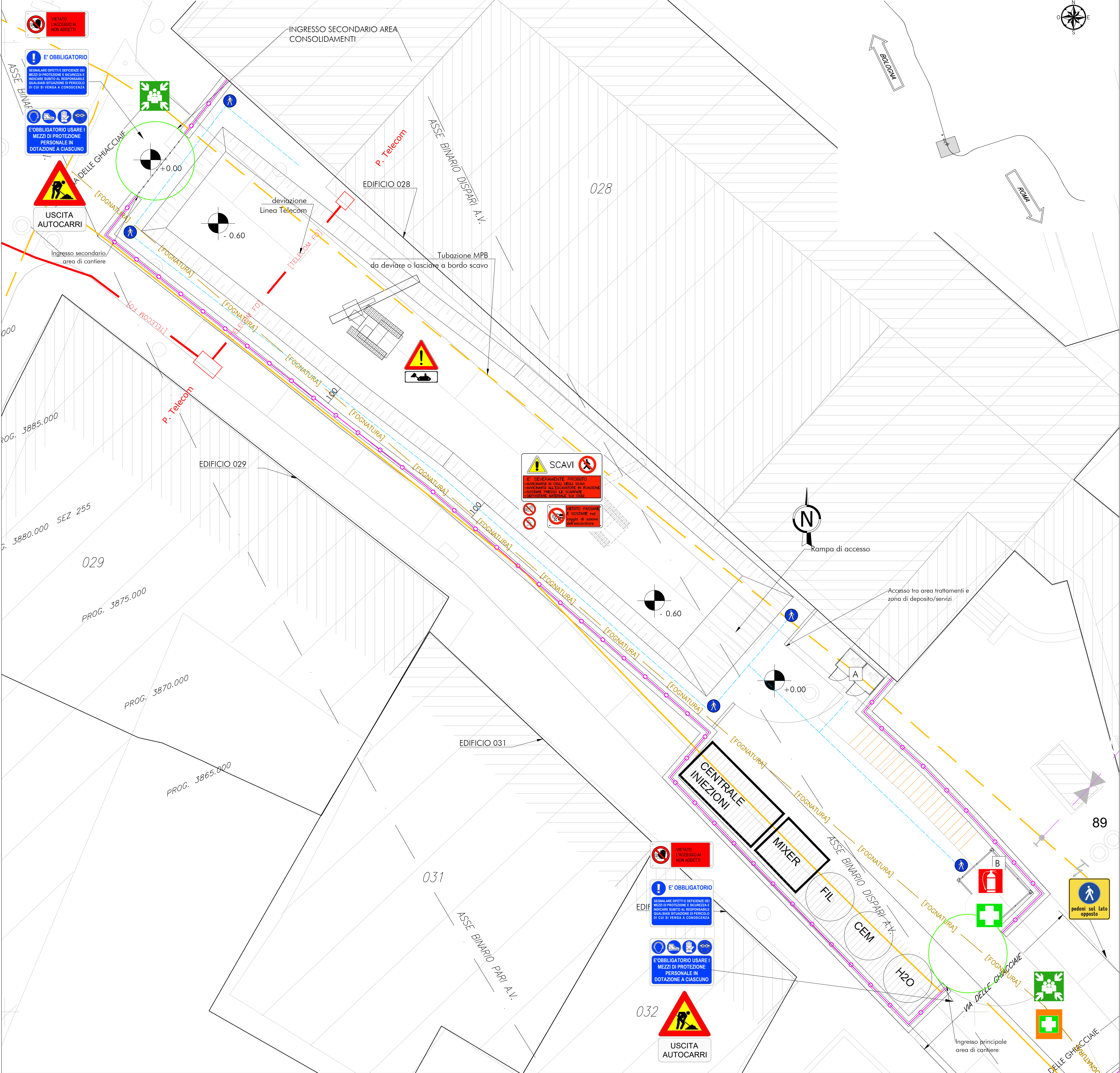
PLANIMETRIA LAYOUT CANTIERE - EDIFICIO 29 scala 1:200
