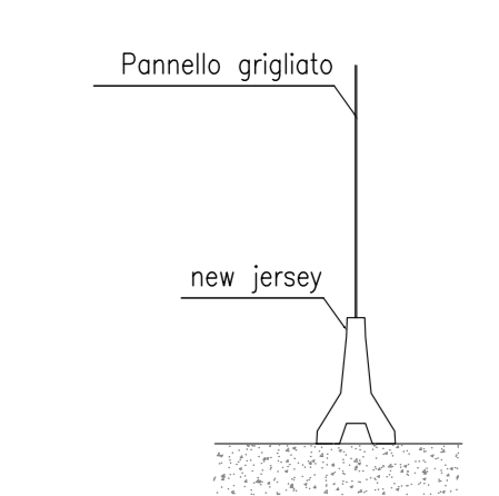
TIPICO RECINZIONE CON PANNELLO GRIGLIATO E NEW JERSEY
