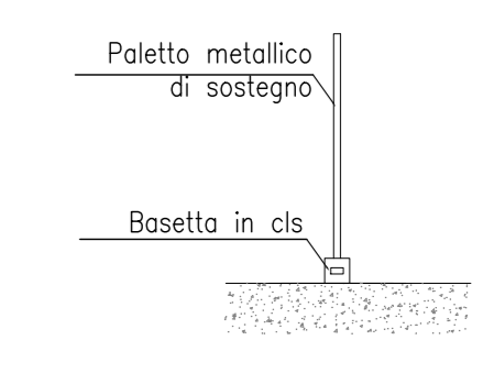
TIPICO RECINZIONE CON PALETTI METALLICI E BASETTE IN CLS
