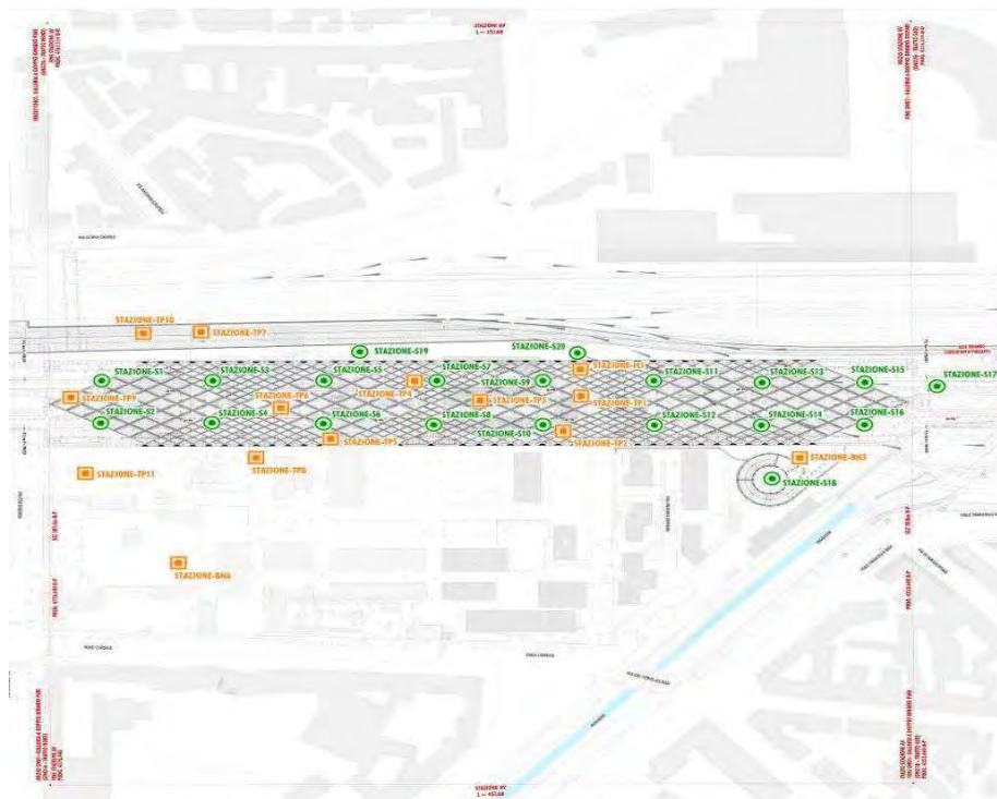
Figura 14. Planimetria con ubicazione dei sondaggi: in giallo i sondaggi eseguiti nel 2005, in verde quelli eseguiti nel 2010
