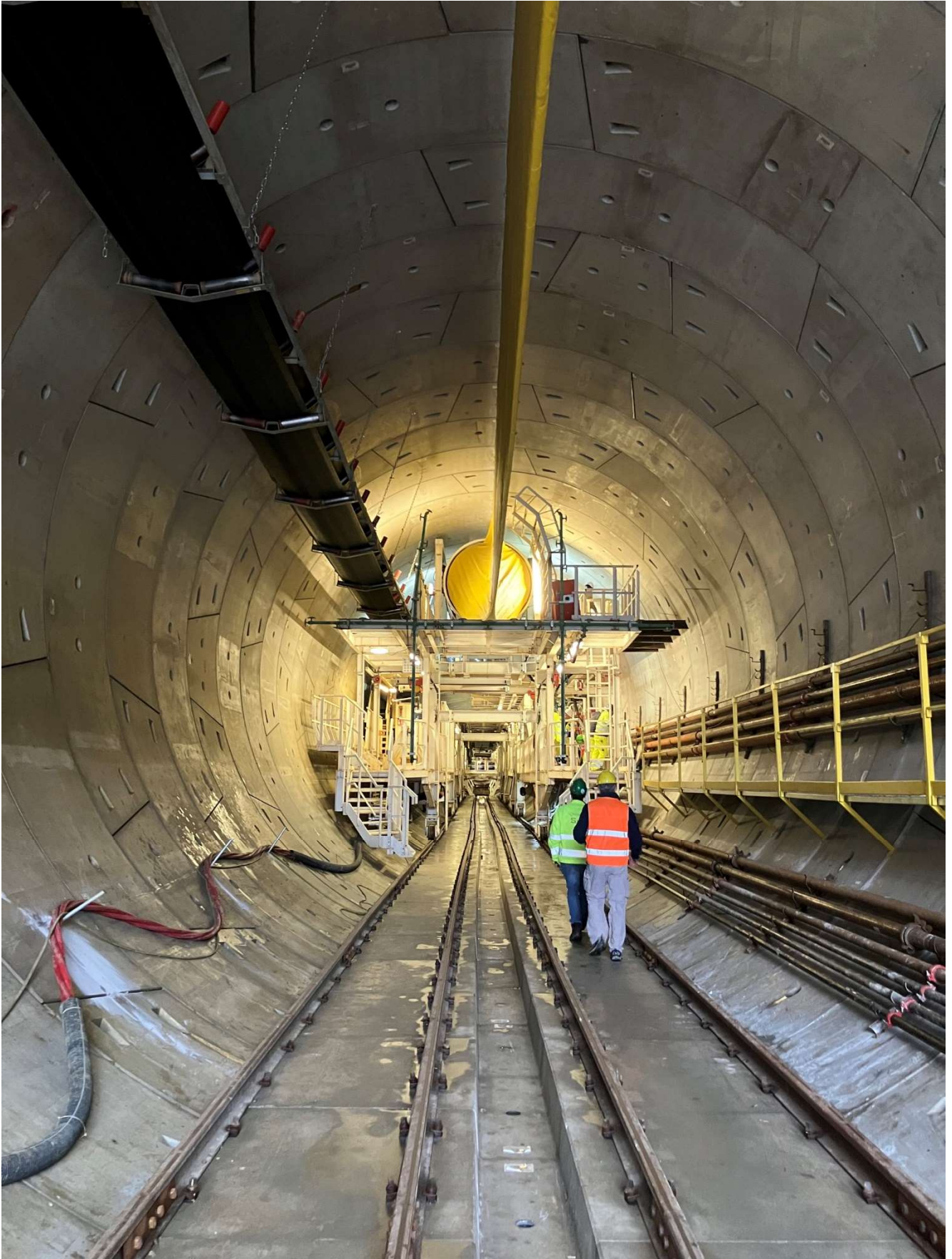
Figura 6 – Scavo Galleria Binario Pari
