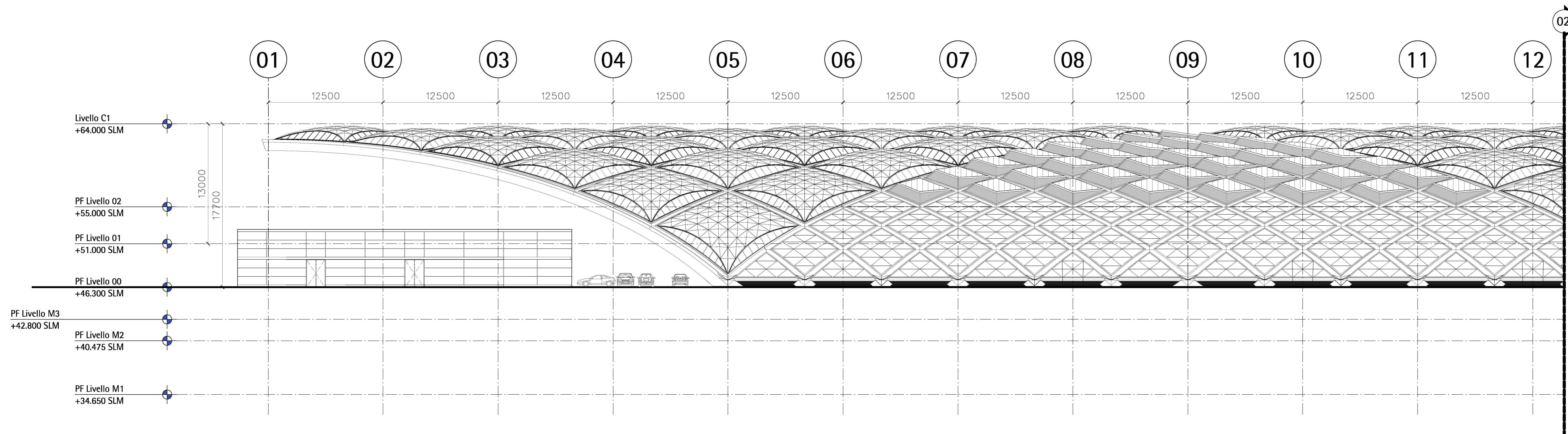
02 (01) Prospetto Ovest 1:200
